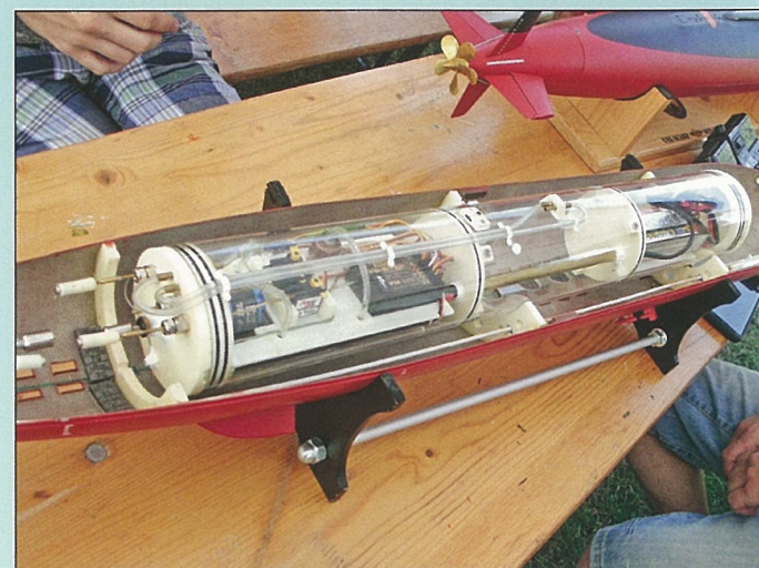
Čistě zpracované a přehledně uspořádané vnitřní vybavení v ponorce Roberta Pokorného
